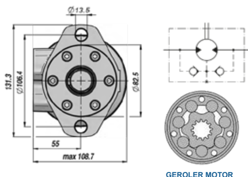
GEROLER MOTOR
